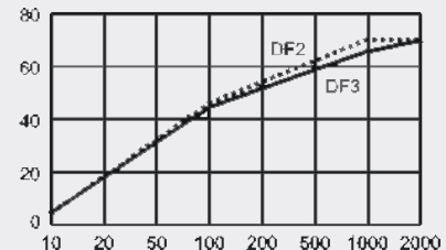
Typische Dämpfungskurve DC-Durchführungsfilter. Typical attenuation DC-feed through filters.
